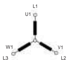
CONNEXION EN ETOILE
