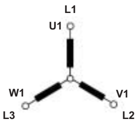
CONNEXION EN ETOILE
