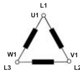
CONNEXION EN TRIANGLE
